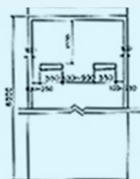
平面配置圖
