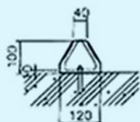
側視圖
