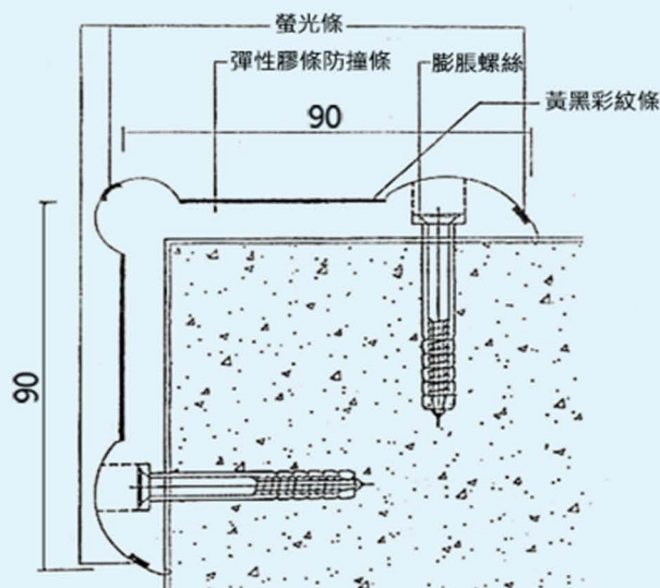
剖面圖
