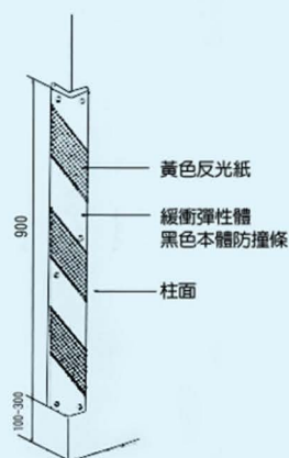
立圖
