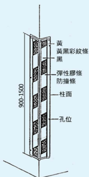
立圖
