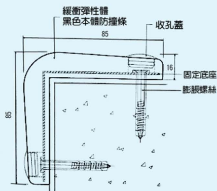
剖面圖
